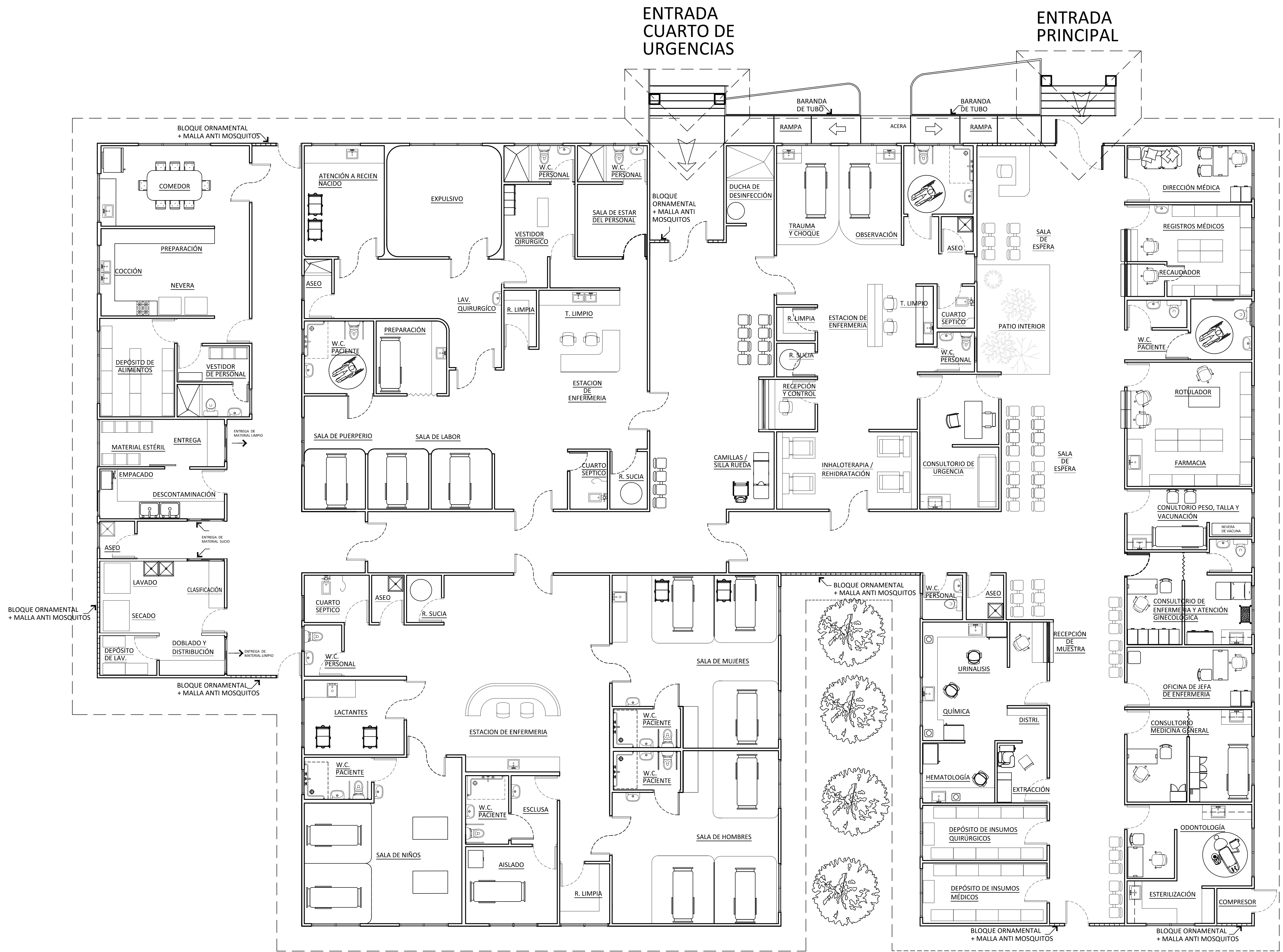
PLANTA ARQUITECTÓNICA - CENTRO DE SALUD DE LAJAS BLANCAS ESCALA 1:75
