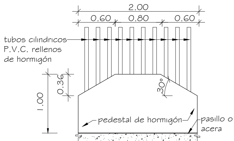
DETALLE DE CERCA EXTERIOR
