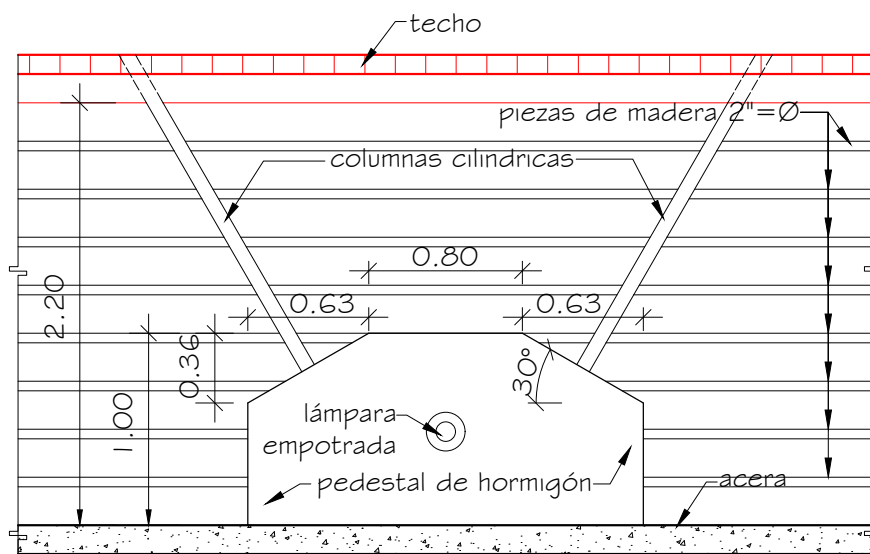
DETALLE DE COBERTIZO-CERCA EXTERIOR
